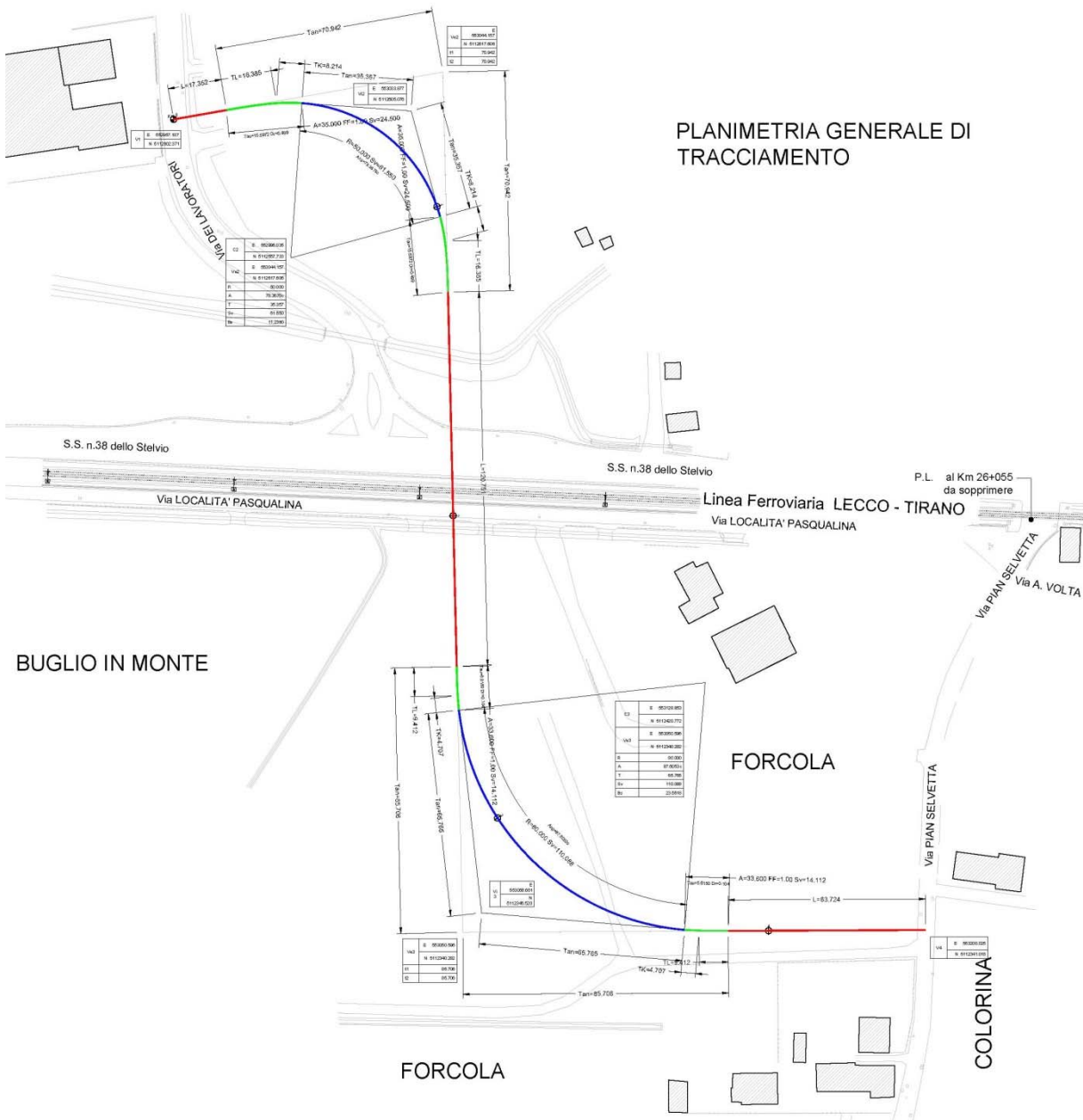
Figura 2.4 – Tracciato planimetrico
